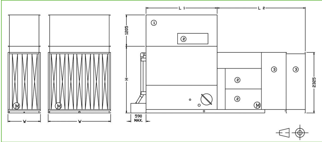
1. Uitlaatdemper; 2. Toegangsdeur; 3. Inlaatdemper; W & H = Toestelafmetingen (Zie Technische gegevens).
