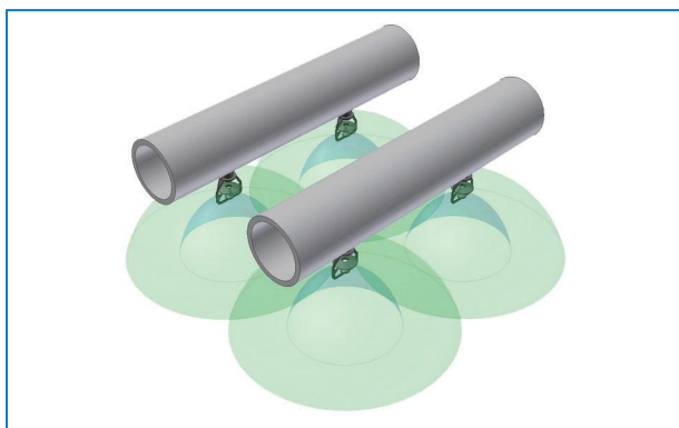
Způsob rozstřiku trysky pro kondenzátor
