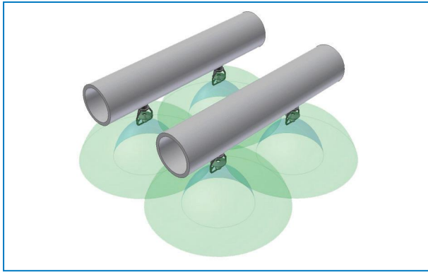
Způsob rozstřiku trysky pro kondenzátor
