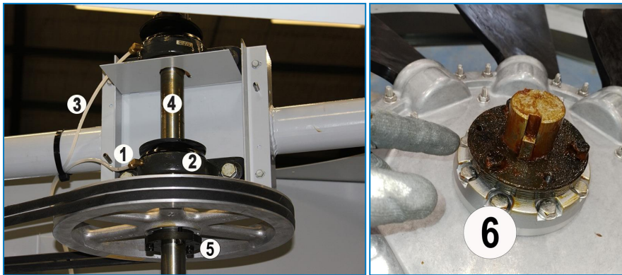
A ventilátortengely-csapágyak és a zsírószemek helye
