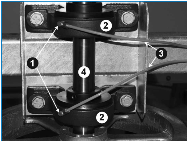
A ventilátortengely-csapágyak és a zsírószemek helye
