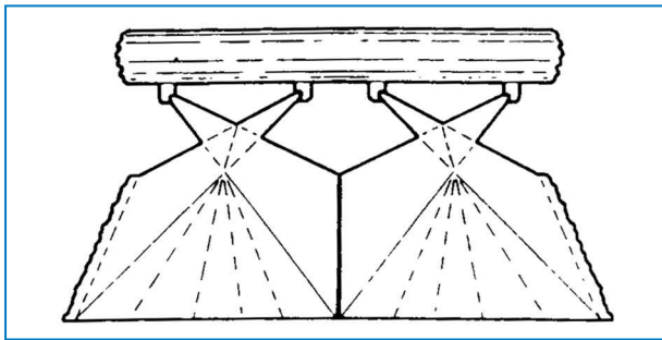
Fúvókás vízelosztású hűtőtorony
