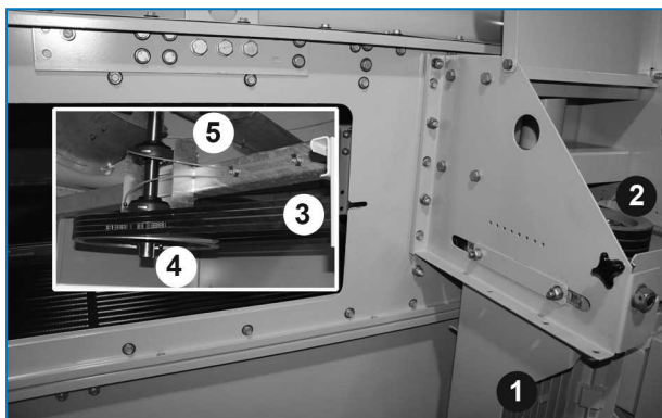
Meghajtó rendszer külső motorral
