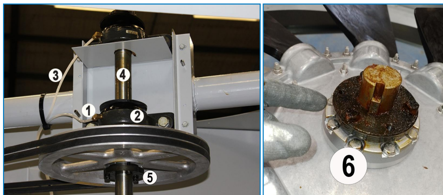
Położenie łożysk wału wentylatora i smarowniczek
