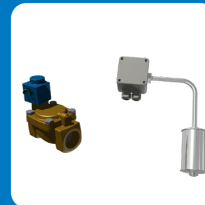
Conjunto del control eléctrico del nivel de agua
