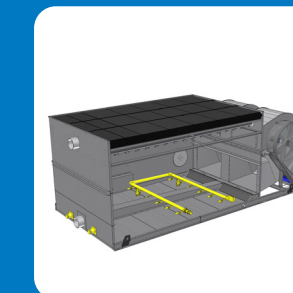
Système d'agitation de bassin
