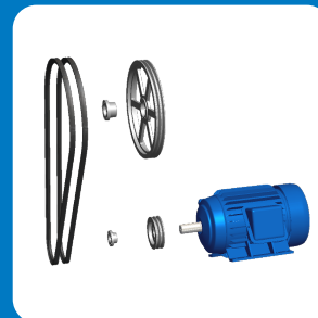
Moteur surdimensionné & Jeu de transmission
