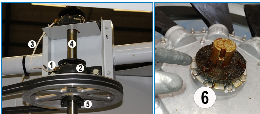
Fläktaxellagers och smörjnippels placering
