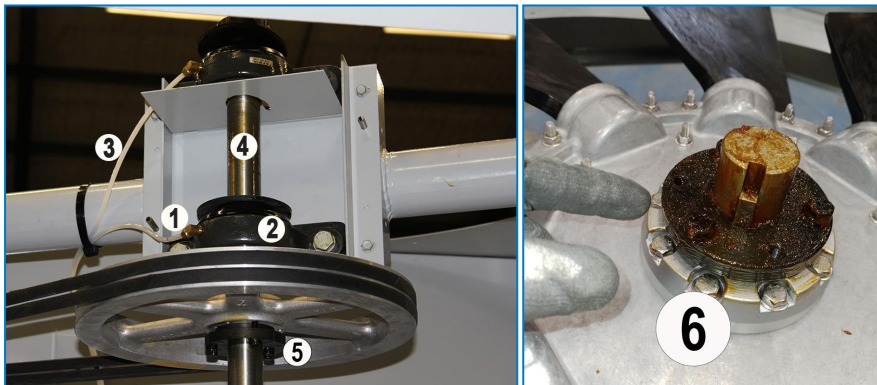
Fläktaxellagers och smörjnippels placering
