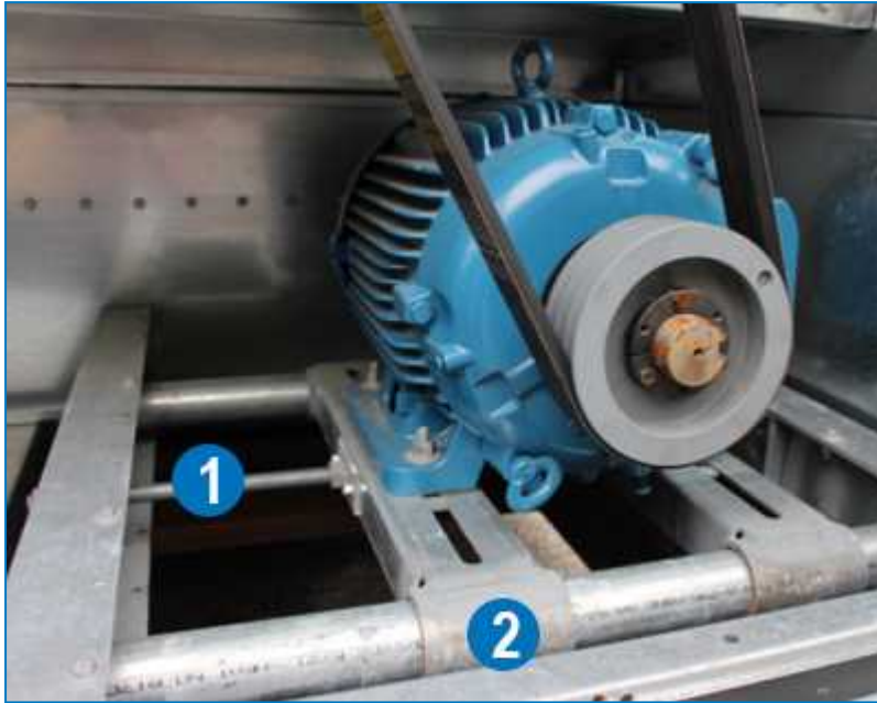
Justerbar motorbas
