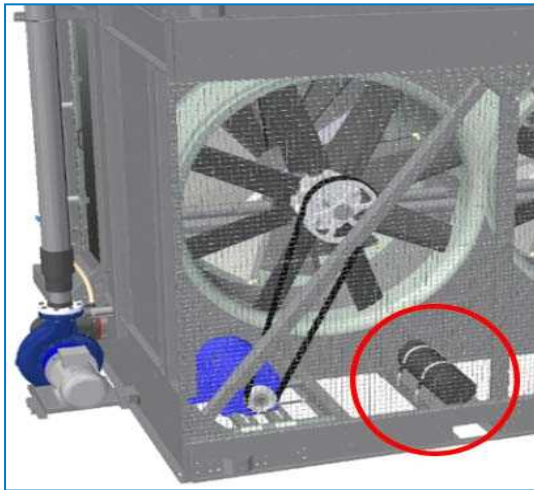
Nödanordningens placering
